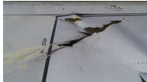
Bild 4: Fragment des Flügels der Boeing 777
